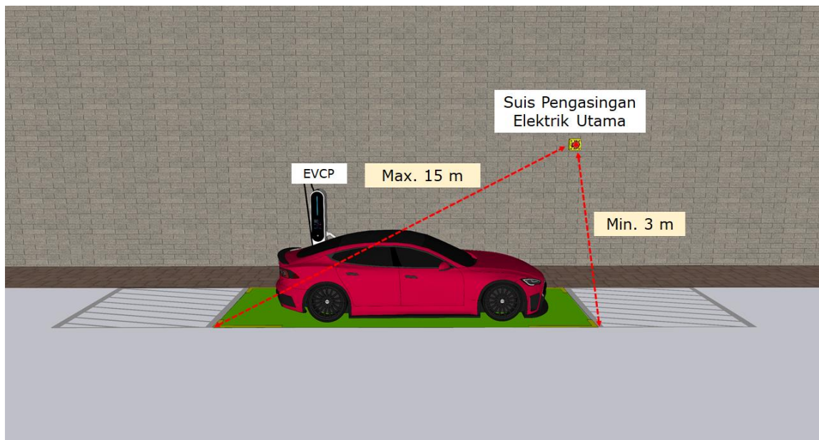
Rajah 11: Perkongsian Penggunaan Suis Pengasingan Elektrik Utama
